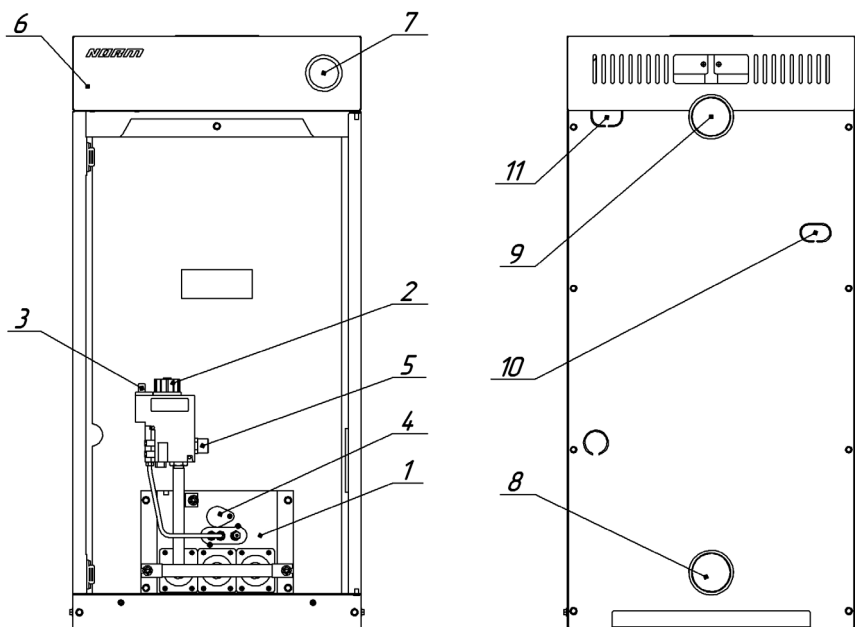
Рис. 1. Котёл «Norm» с автоматикой 630 EUROFIT
